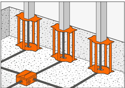
Sternverdrahtung: Erd-Abzweigkasten star wiring: earth distribution box
