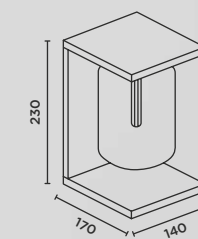
Größe in mm size in mm
