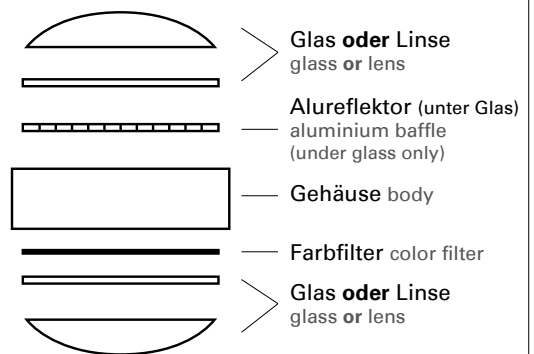
Puk Meg Maxx Kopfkfiguration (frei wählbar) Puk Meg Maxx Configuration (freely selectable)
